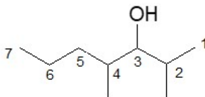
2,4-diméthylheptan-3-ol
